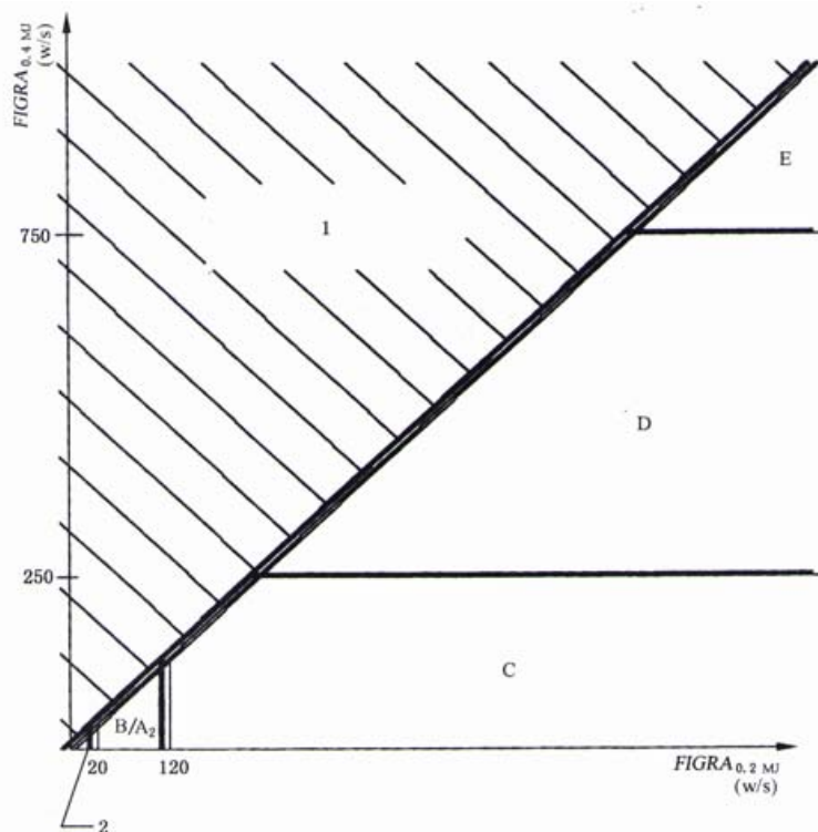
图 A.1 表 1 中定义的等级和 ISO 9705: 1993 试验结果之间的关系
